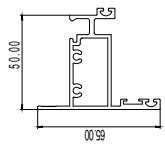
TJ741 50 H/D AW Sash
