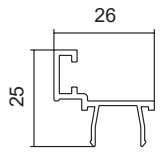
TJ706 45mm Door Stop
