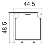
TJ200 Pivot Stile
