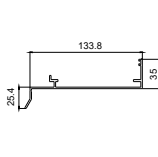
TJ259 Sub Sill 23mm S.Back
