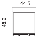
TJ201 Hinge Stile/Plain
