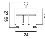
SWD419 Patio Door Fly Door Raised Clip-on Track
