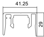
SWD038 Patio Door STD Interlock W' Flydoor Interlock Attached
