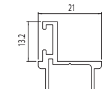
CSG335 35mm Door Stop
