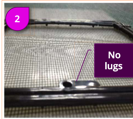
No lug goes under screen
