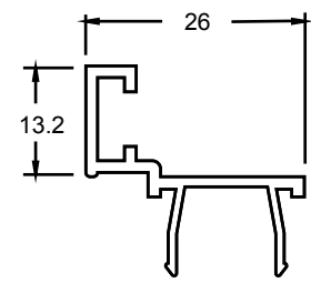
TJ706 45mm DOOR STOP
