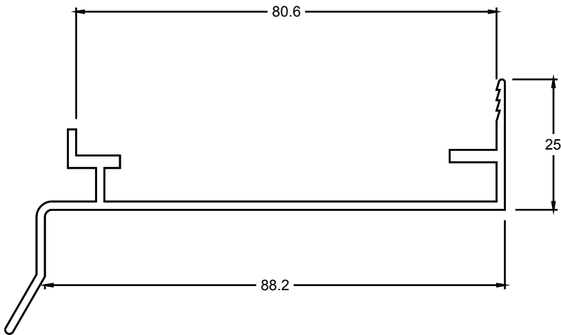
TJ759 SUB SILL
