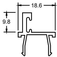
TJ735 35 mm DOOR STOP
