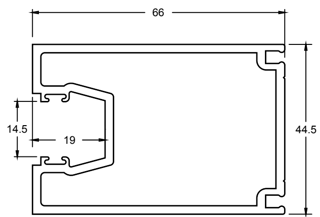
HV271 DOOR STILE
