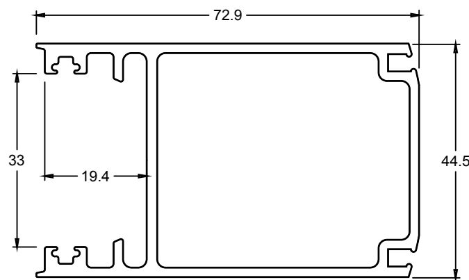
TJ421 PIVOT STILE
