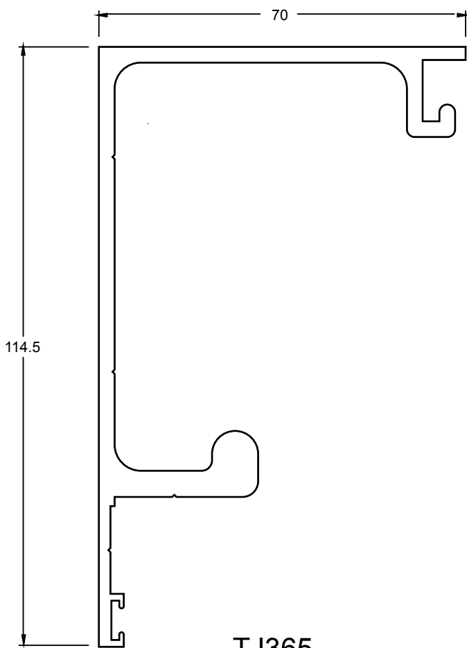
TJ365 H/D DOOR TRACK
