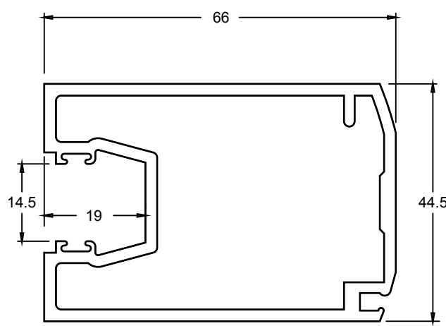
HV312 LOCK STILE
