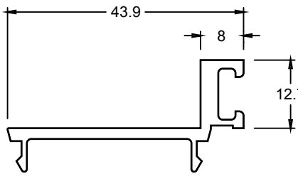
CDG6507 DOOR STOP
