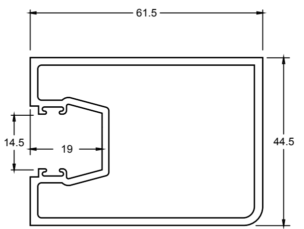
HV272 HINGE STILE
