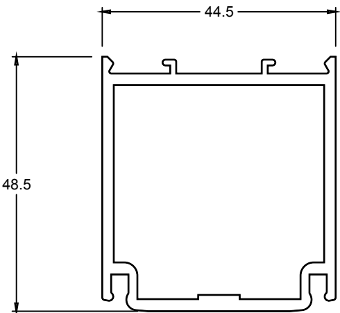
TJ200 PIVOT STILE
