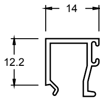
TJ202 DOOR BEAD
