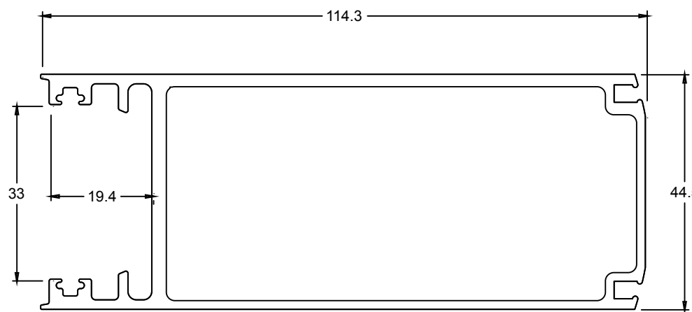
TJ439 PIVOT STILE
