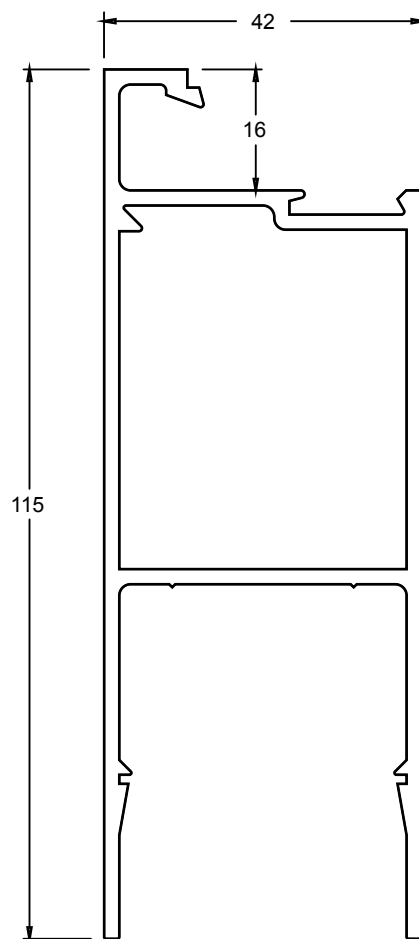
TJ315 DOOR BOTTOM RAIL
