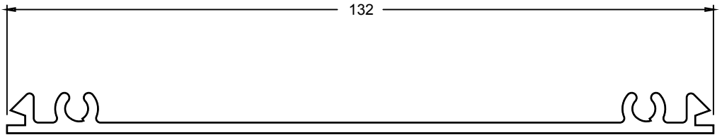
JM2865 FLAT FILLER
