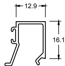
HV274 DOOR BEAD
