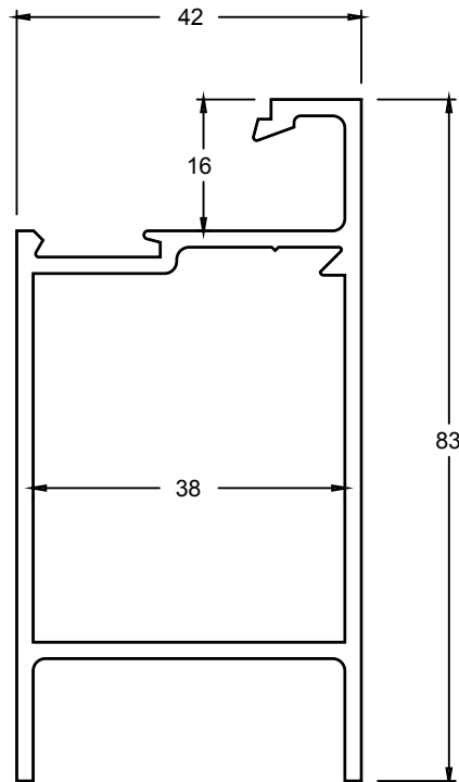
TJ313 DOOR TOP RAIL
