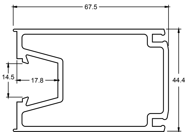
TJ321 PIVOT STILE
