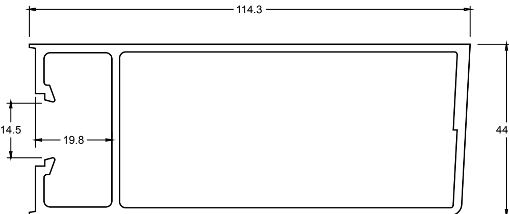
TJ451 HINGE STILE
