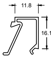
TJ314 DOOR BEAD
