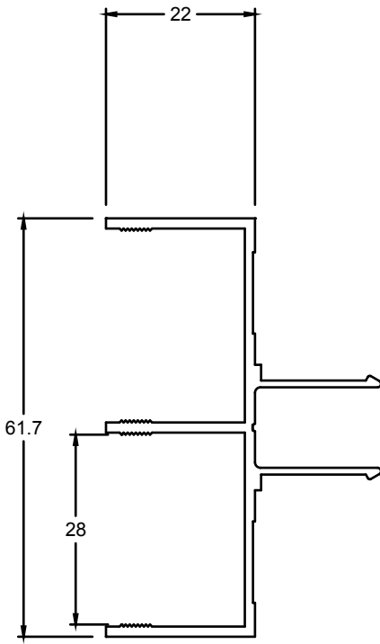
DH108 JAMB INSERT
