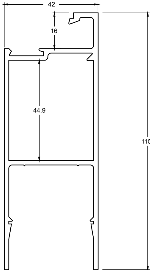
TJ315 DOOR BOTTOM RAIL
