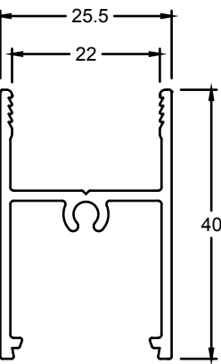
DH255 STILE DG
